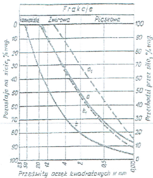
Rysunek 1. Obszar uziarnienia optymalnych mieszanki żwirowej.
